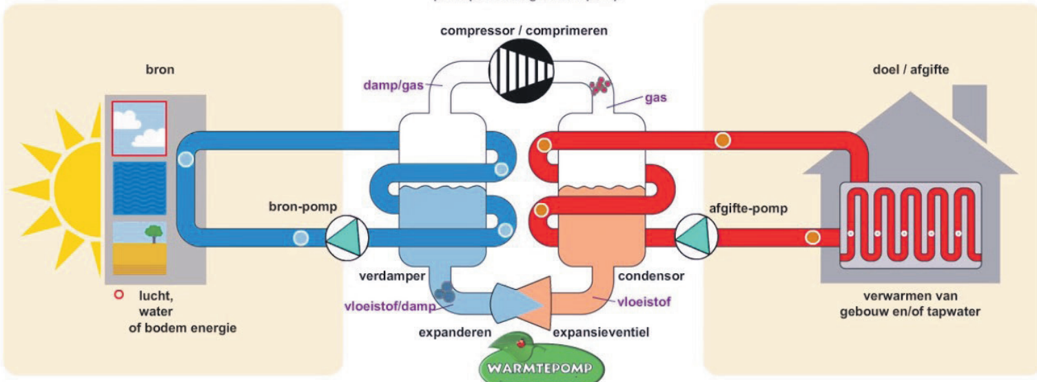
principe werking warmtepomp
